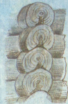
Рубка „в обло“ (чашкой вниз).
